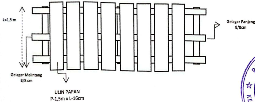
GAMBAR TAMPAK ATAS
