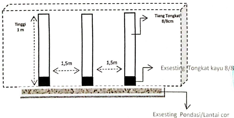
GAMBAR TIANG ULIN PENGUAT RANGKA
