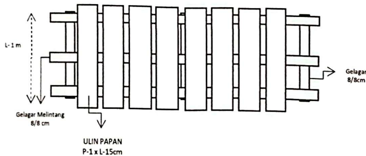
GAMBAR TAMPAK ATAS
