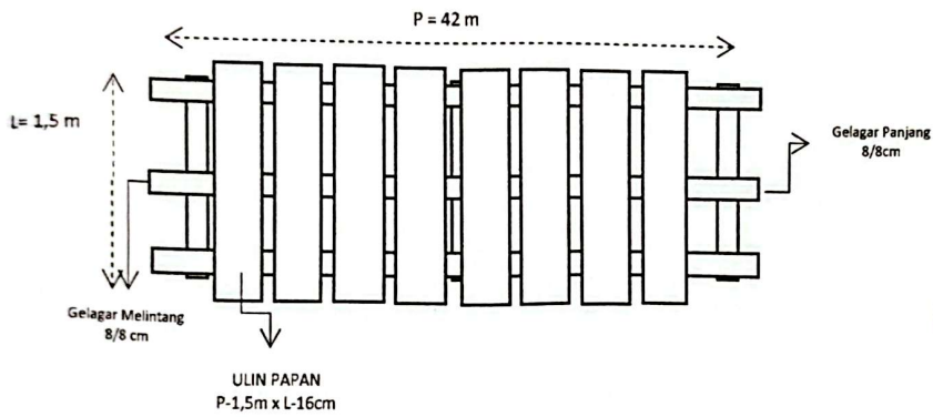
GAMBAR TAMPAK ATAS
