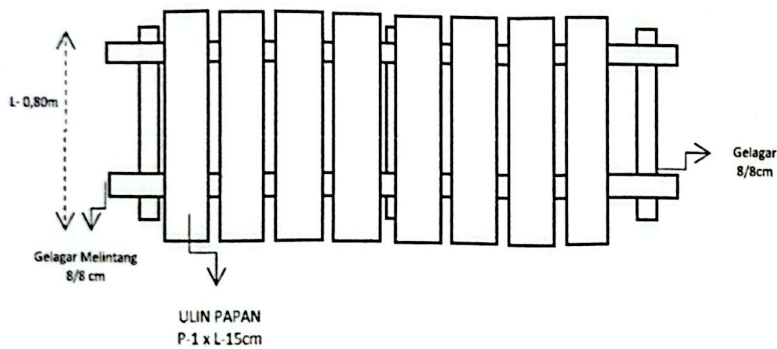
GAMBAR TAMPAK ATAS
