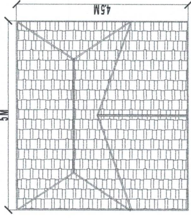
BANGUNAN TAMPAK ATAS
