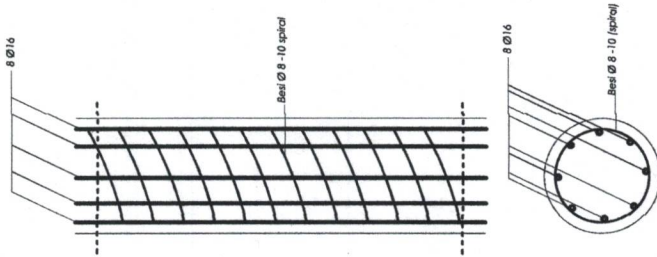
KOLOM Ø 40 Skala 1 : 10
