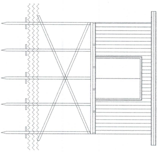
BANGUNAN TAMPAK DEPAN
