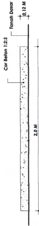
DETAIL POTONGAN A-A
