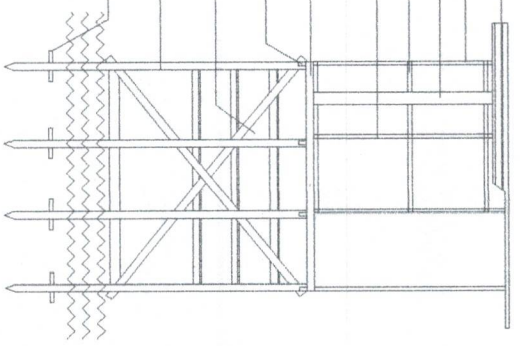
BANGUNAN TAMPAK SAMPIING 1
