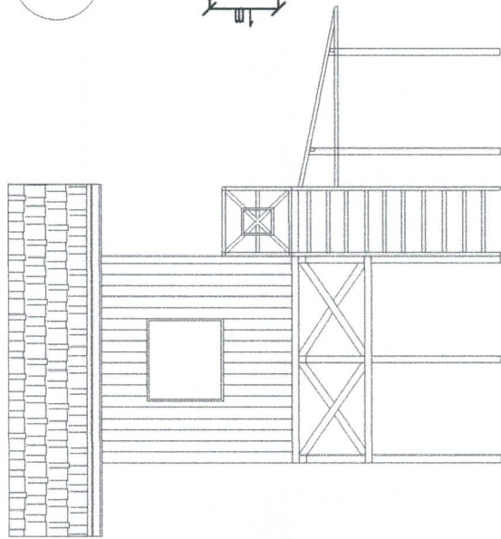
BANGUNAN TAMPAK SAMPING
